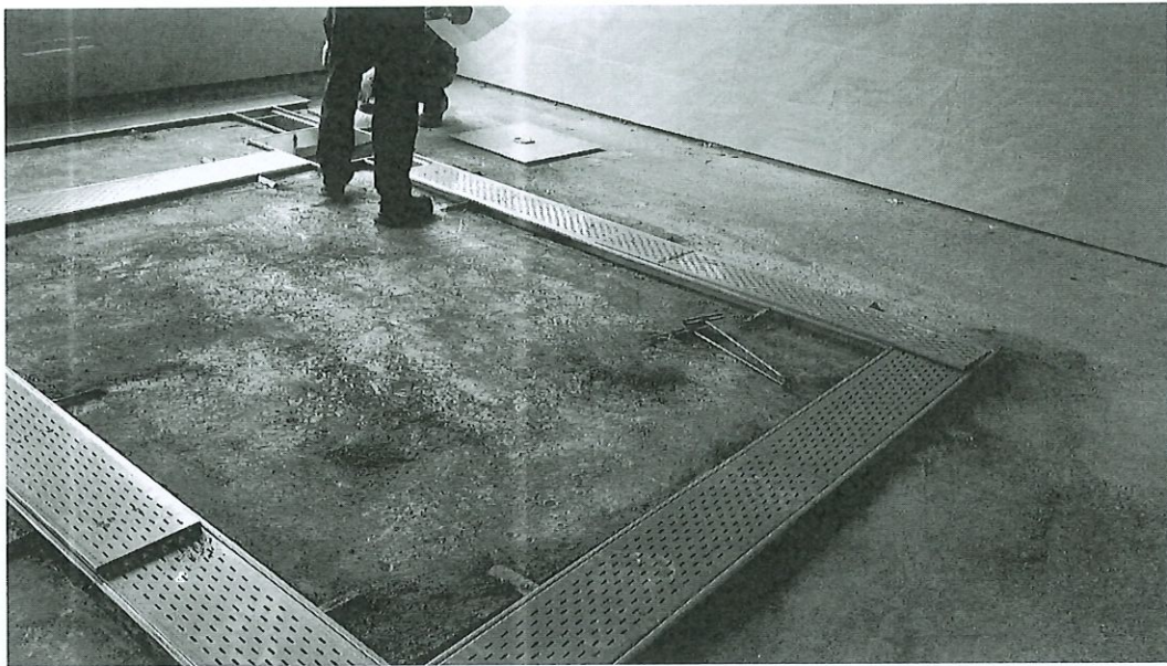
廚房截水溝
